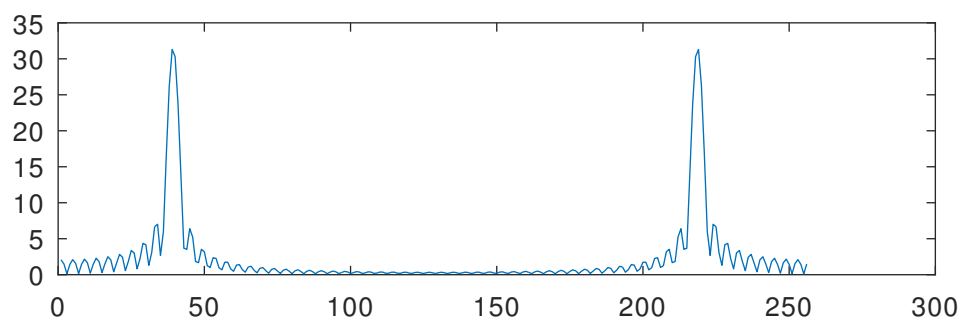
FFT sem Janela (Vazamento espectral alto)
